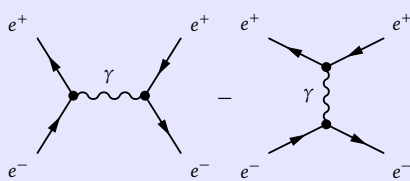
Bhabha 散射 e^+e^- \rightarrow e^+e^-
