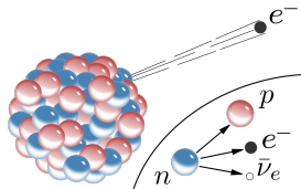
原子核 \beta 衰变
