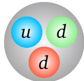
中子
