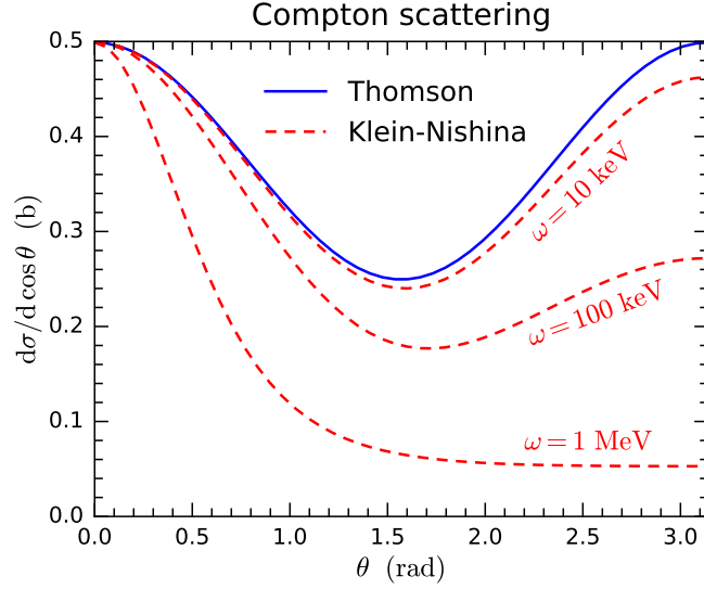
图 8.13: Thomson 公式和 Klein-Nishina 公式给出的微分散射截面随散射角 \theta 的变化。
