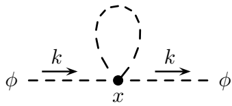
图 7.12: iI_2^{(1)} 贡献的 \phi 粒子自能图。
