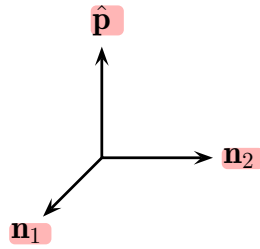
图 3.10: 单位矢量 \hat{\mathbf{p}} 、 \mathbf{n}_1 和 \mathbf{n}_2 示意图。
